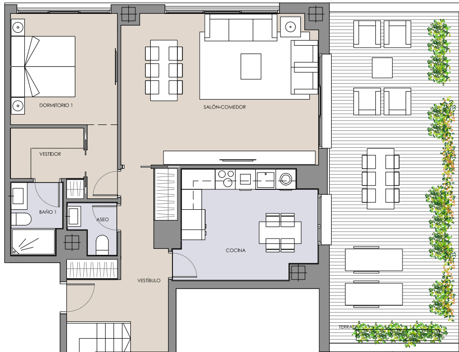
PLANTA ÁTICO
