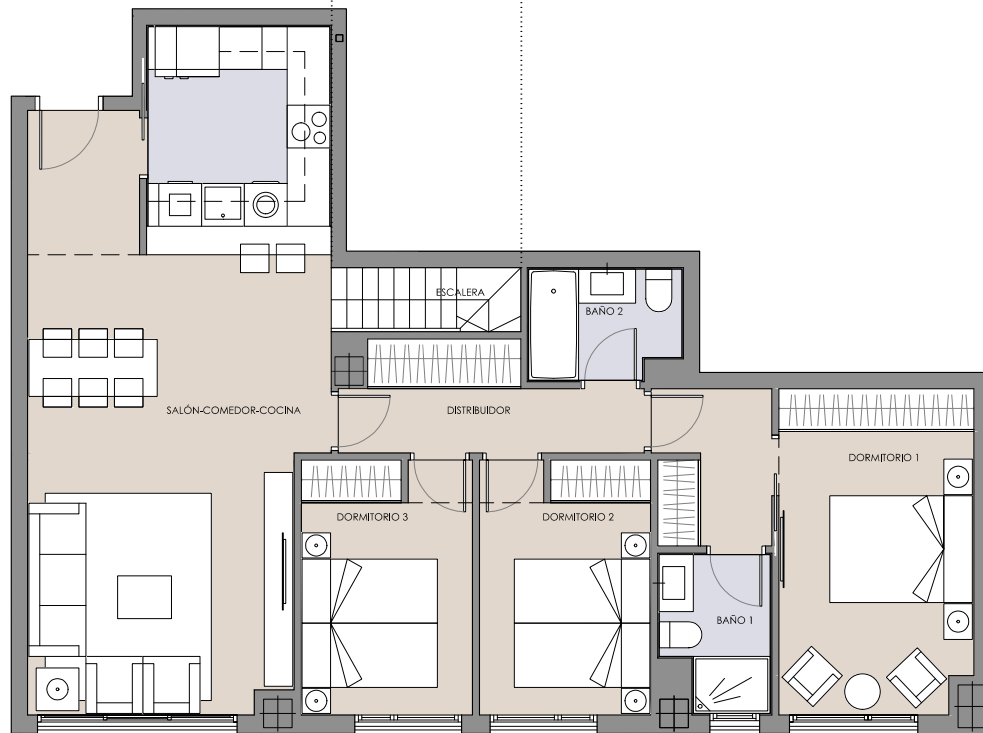
PLANTA SEXTA
